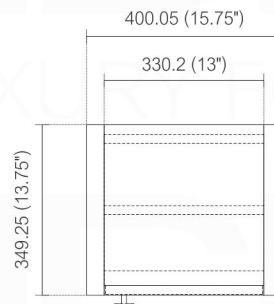
. TOP ELEVATION
