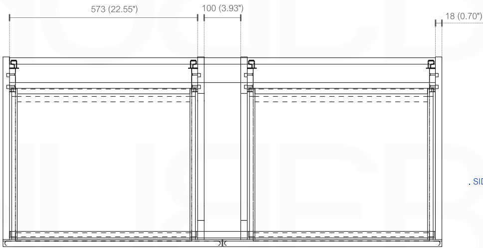
. TOP ELEVATION
